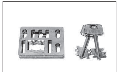
Juego de gorjas Para cerradura persiana metálica "6511" 2 llaves.
