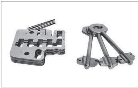
Juego de gorjas de 4 vueltas con 3 llaves. Código: JU000001
