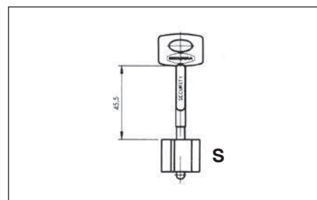
Llave larga de 45,5 mm EZCU4100S
