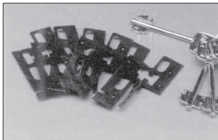
Juego de gorjas de 2 vueltas
